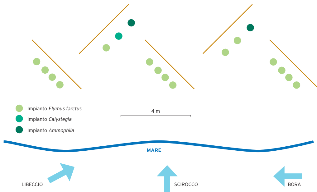
Figura 10: schema indicativo di della configurazione di intervento finalizzata allo sviluppo di dune embrionali, con l'impiego di strutture frangivento alte 50 cm e impianto di vegetazione (la distanza dal mare non è in scala) (elaborazione propria).
