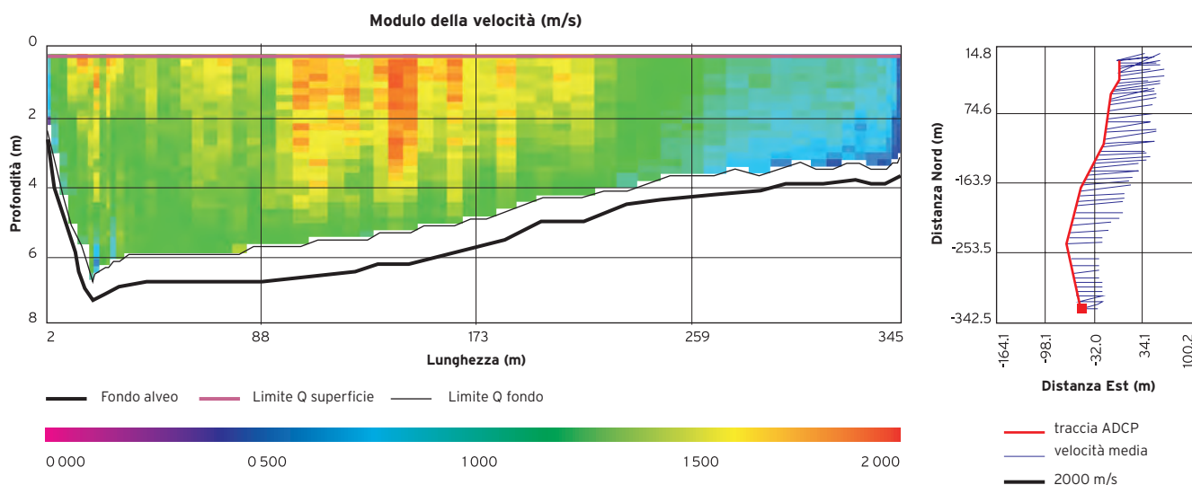
Figura 3: misura effettuata con ADCP sulla sezione S4-b (Po di Pila) il giorno 06/11/2010 dalle ore 10.57 alle 11.02: a destra è riportato il percorso eseguito e a sinistra il grafico di distribuzione delle velocità.
