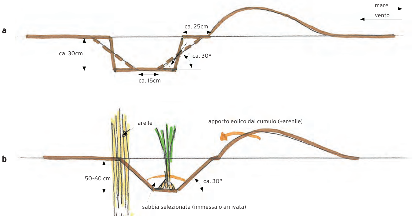
Figura 7: esempio di impianto di Ammophila nell'alto arenile. Fasi di impianto (a, b) e sviluppi attesi (c,d). In marrone scuro, profilo delle sabbie da rifluimento presenti al momento dell'impianto; in marrone chiaro, profilo delle sabbie classate di apporto eolico.
