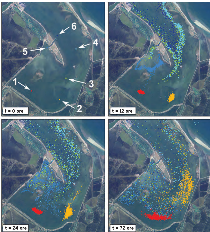
Figura 1: Illustrazione del processi dispersivi subiti da sei macchie immerse nella parte meridionale della laguna di Vallona.
