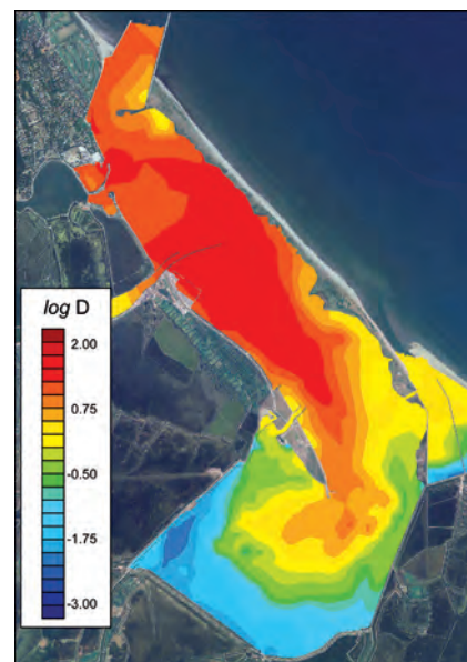
Figura 2: distribuzione spaziale del logaritmo del coefficiente di dispersione intermareale, D espresso in m^2/s . (laguna di Vallona).
