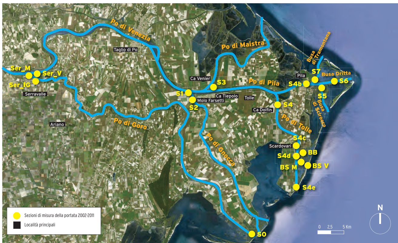
Figura 1: inquadramento delle sezioni di misura ubicate sui principali rami del Delta.
