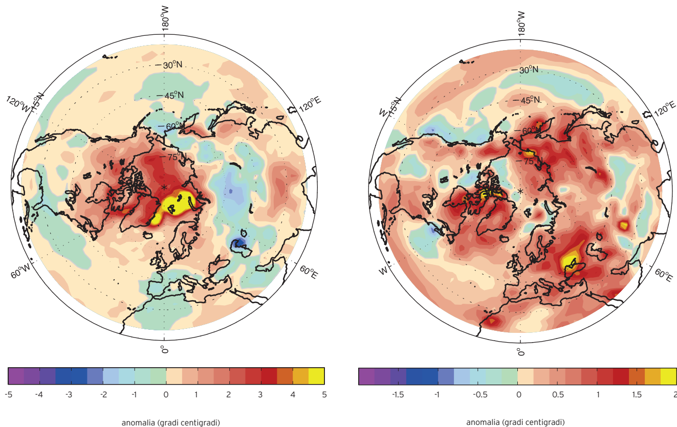
Anomalie di temperatura dell'aria periodo 2005-2010, DGF
